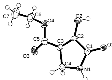
Abb. 2. Molekülstruktur von Ethyl-3-hydroxy-2-oxo-3-pyrrolin-4-carboxylat ( 21 ) im Kristall (Auslenkungsellipsoide mit 50 % Aufenthaltswahrscheinlichkeit, Wasserstoffatome mit willkürlichen Radien). Ausgewählte Bindungslängen [Å] und -winkel [°]: C1–O1 1.247(4), C2–O2 1.326(4), C1–C2 1.492(4), C2–C3 1.342(4), C3–C4 1.503(5), C4–N1 1.453(4), N1–C1 1.316(4); O3–C5–O4 125.2(3), O4–C6–C7 110.9(3).
